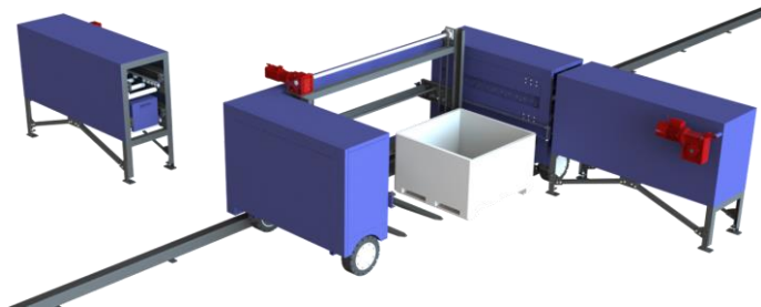
Carro eléctrico autónomo para el traslado de bins con su set de baterías de carga automatizada
